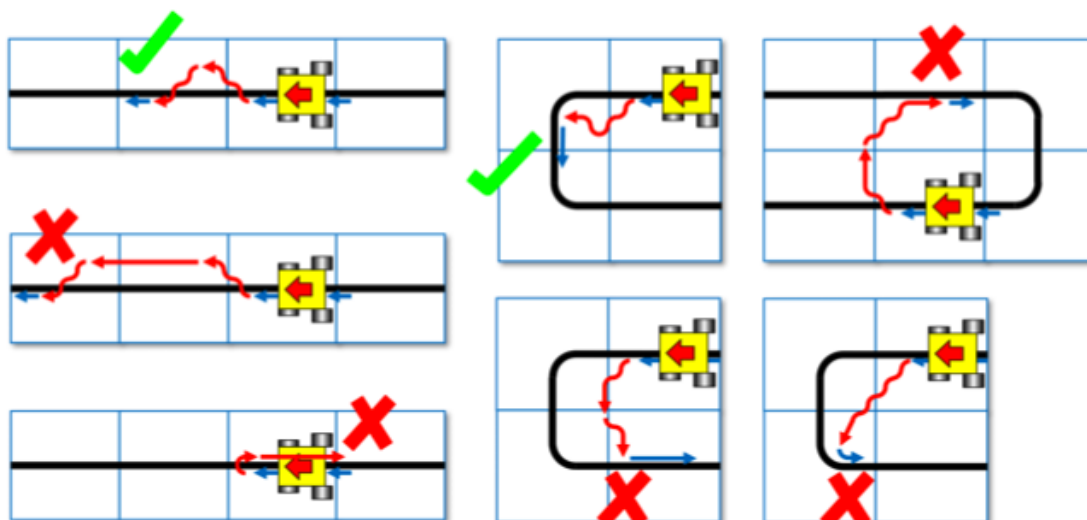
Рис.7. Примеры потери роботом линии.
