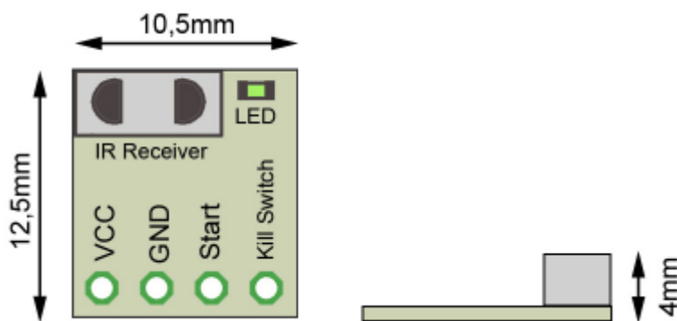
Рисунок 2. Пример модуля
