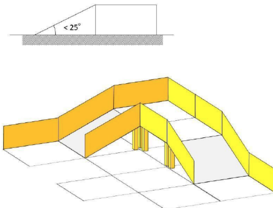
Рис. 2. Внешний вид пандуса
