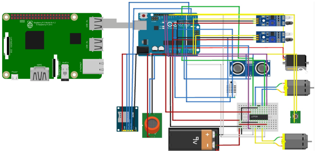
Рисунок №1 “Схема на макетной плате”
