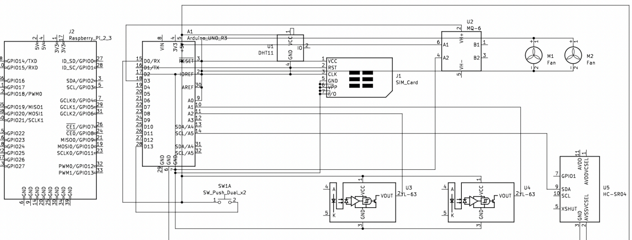
Рисунок №2 “Принципиальная схема”
