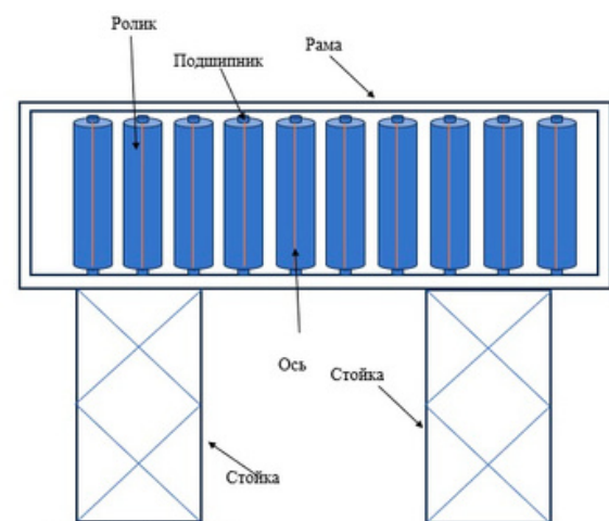
Ролиганг и манипулятор с захватом
