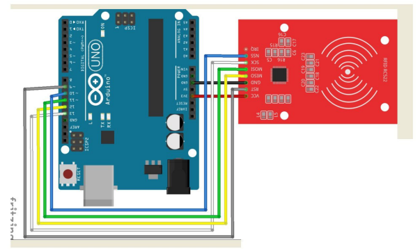
Схема стационарного считывателя
